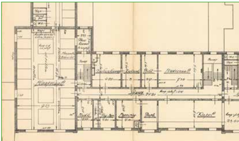
Afb. 2 Plattegrond van de voorbouw van het fraterklooster Anno 1924 (Reg. Archief Tilburg, nr 747, n° 2)
